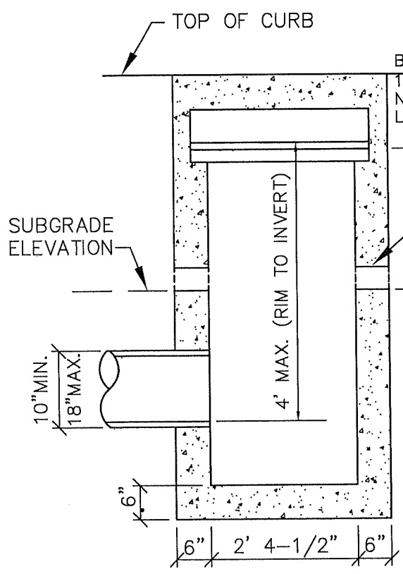
SECTION A-A
