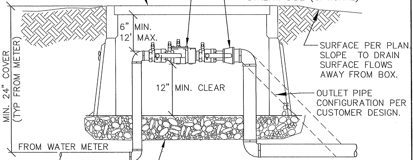
ELEVATION
